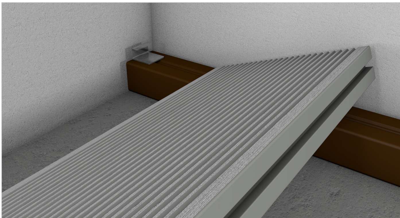
Rys 14. Montaż pierwszej deski na klipsie startowym
