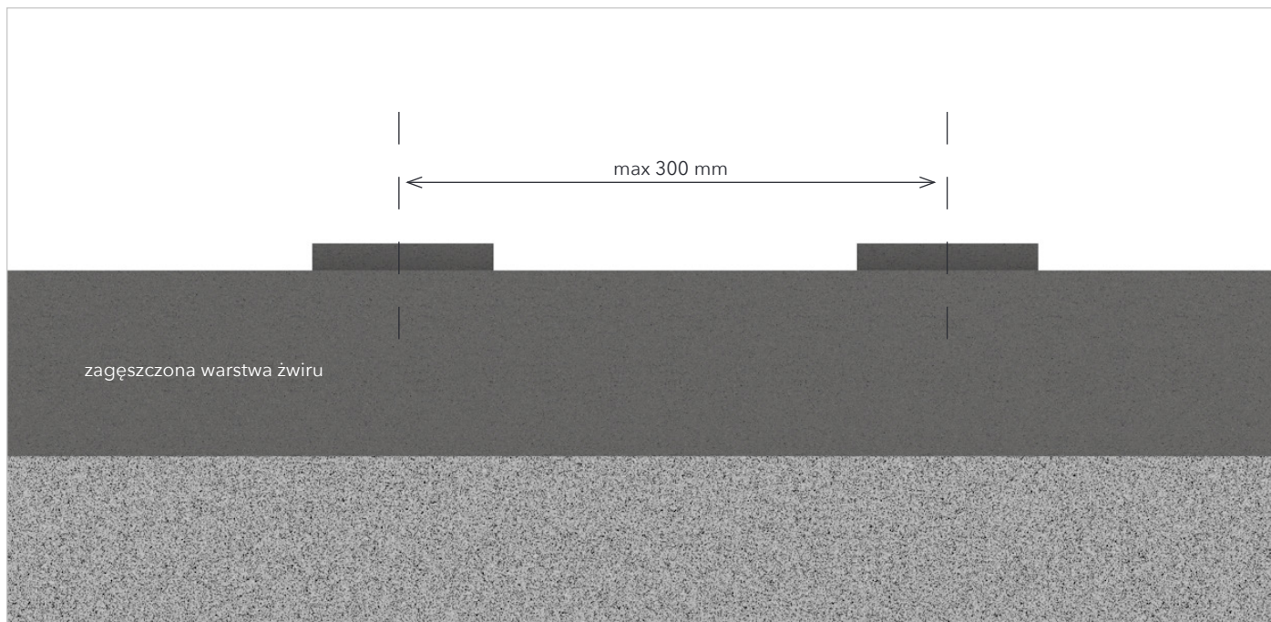
Rys 6. Podłoże na gruncie - taras na płytach betonowych
