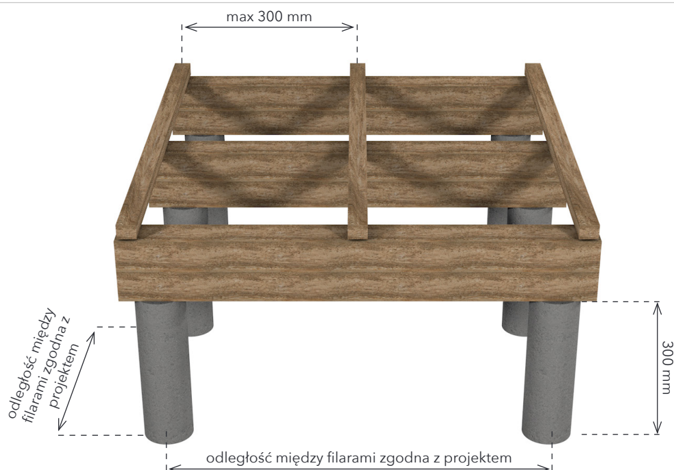
Rys 5. Podłóże na gruncie - taras na podporach betonowych i kantówkach o większej nośności niż legar WPC
