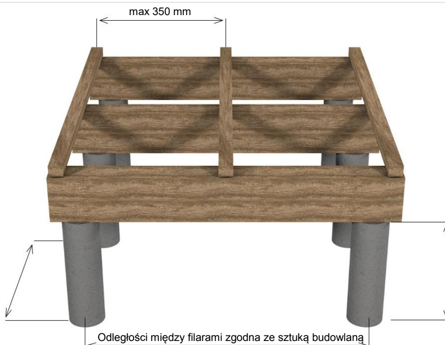
Rys 5. Podłoże na gruncie - taras na podporach betonowych i kantówkach o większej nośności niż legar WPC
