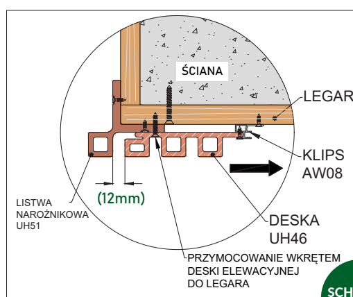
SCHEMAT 21-2
