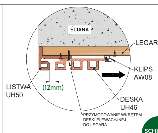
SCHEMAT 21-1
